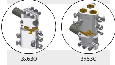
TRAFCONNECT 3 WAY 630
